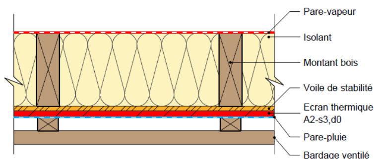
ITEP – F3 - isolant en âme – voile de stabilité intérieur - écran thermique laine de roche
