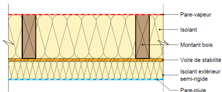
FOB 3 – isolant en âme et complément d'isolant extérieur
