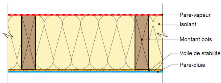
FOB 3 – isolant en âme et complément d'isolant extérieur
