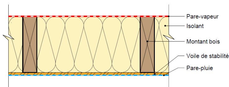
FOB 2 – isolant en âme et complément d'isolant intérieur
