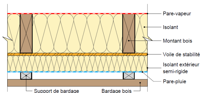
FOB 3 – isolant en âme et complément d'isolant extérieur
