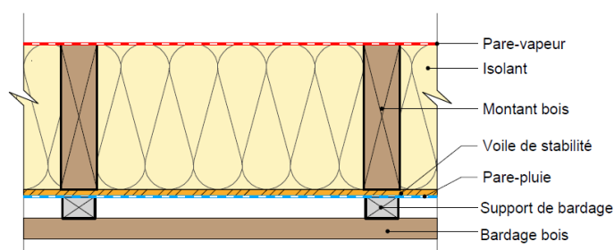
FOB 1 – isolant en âme
