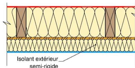
Mur 7 : isolant en âme et ITE avec finition enduit
