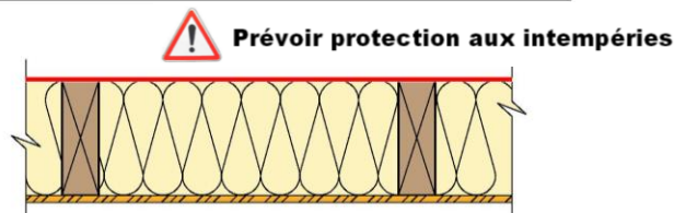
Mur 7 : isolant en âme et ITE avec finition enduit
