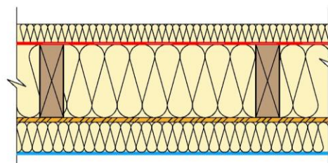
Mur 8 : isolant en âme et en doublage intérieur et extérieur
