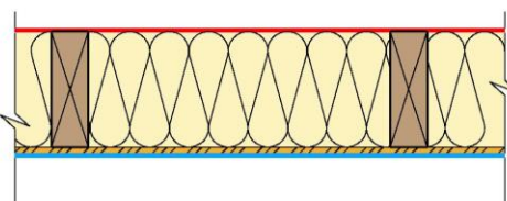
Mur 6 : isolant en âme et en doublage extérieur
