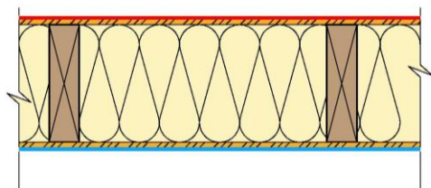
Mur 4 : isolant en âme et en doublage intérieur
